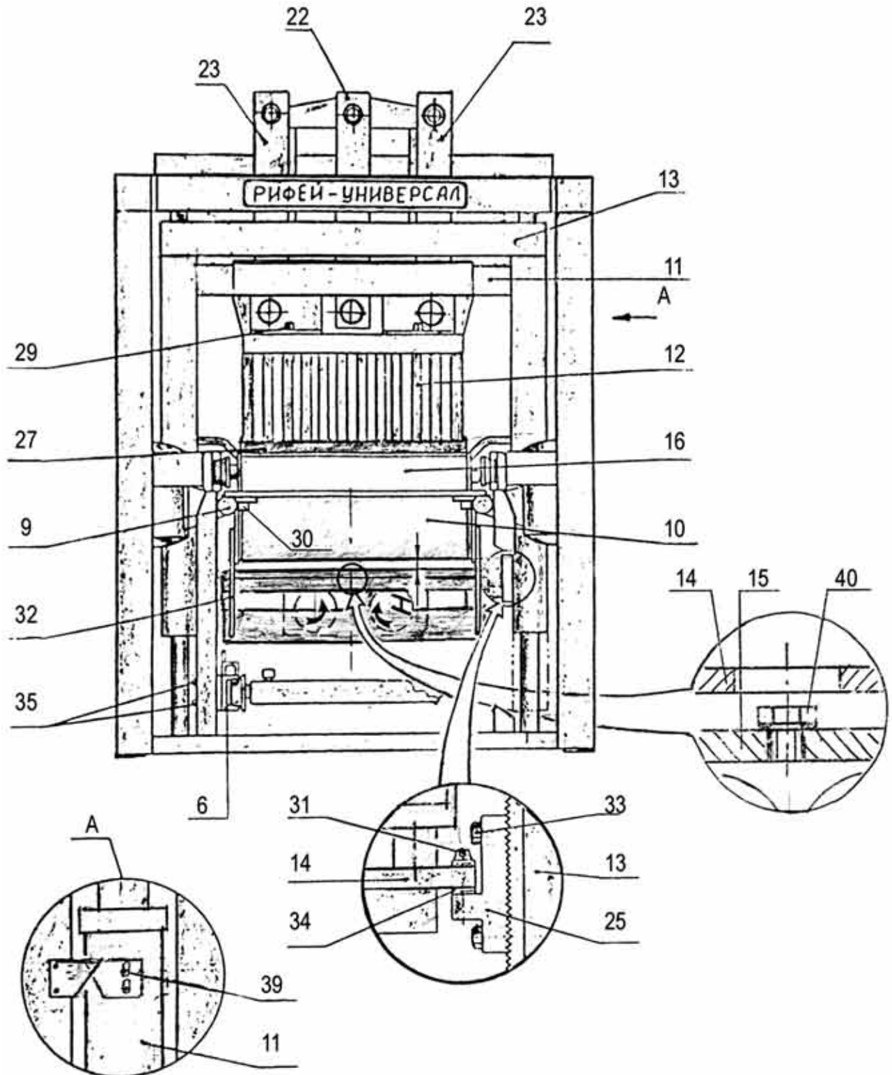
Рис 5 б. Вибропресс.
