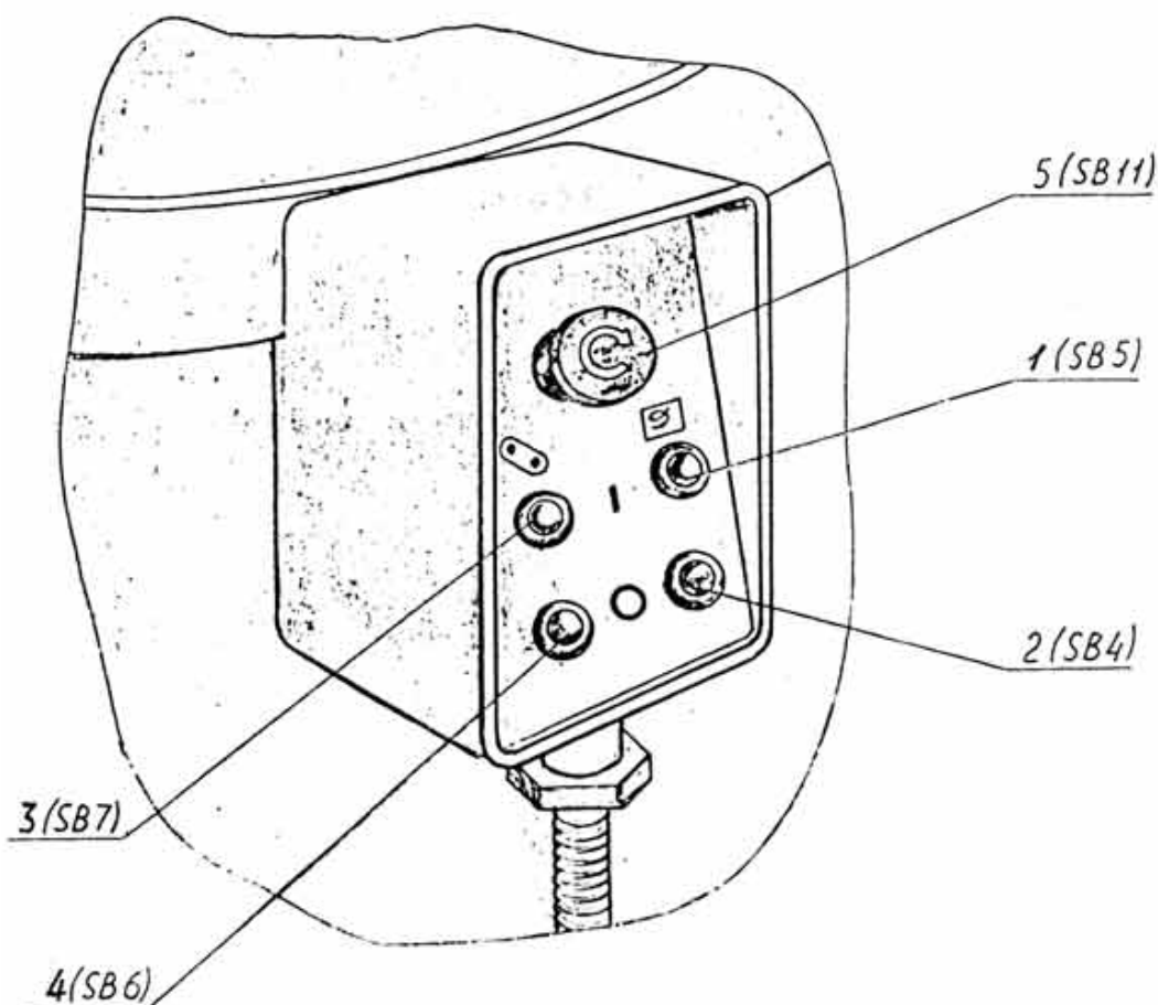
Рис. 13. Пульт управления смесителем и транспортером
