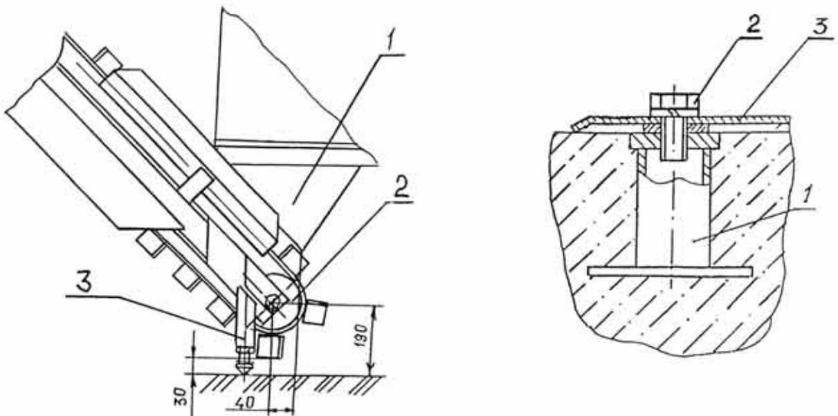
Рис. 18 1-бункер вибропресса; 2-рама вибропресса; 3-кронштейн транспортера; 4-крепежный болт; 5-дефлектор;
