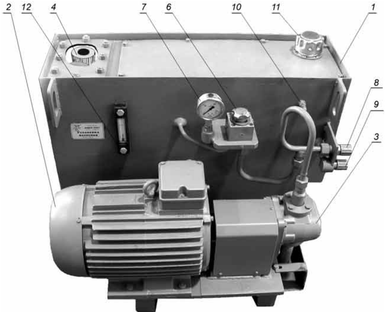
Рис. 8 Насосная установка
