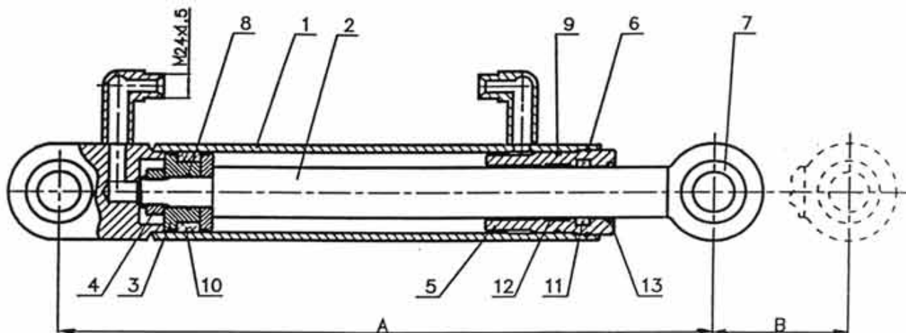
Рис. 10. Гидроцилиндр
