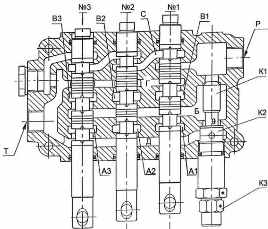
Рис. 9. Гидрораспределитель HC-D10/3
